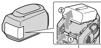
Tlačidlo PUSH (uvoľnenie batérie)
