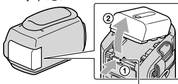
Uvolňovací páčka PUSH (uvolnění akumulátoru)
